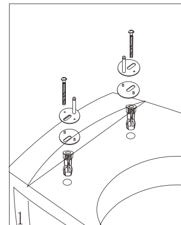
Monteer alle onderdelen
