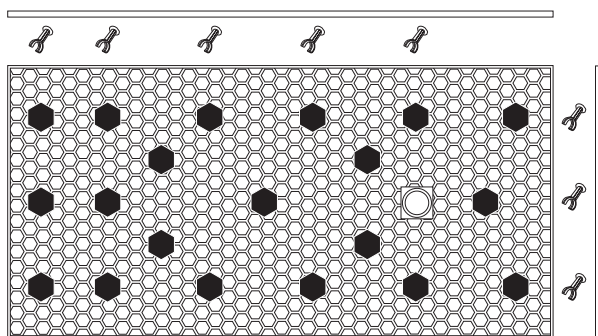
Aanbevolen positie van de U-pootjes.
